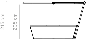
Kosmos shade rond haute + Kosmos 8-places
