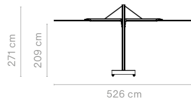
Diamant quattro + socle à roulettes
