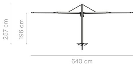
Carré duo + fixation permanente & l'extension du mât
