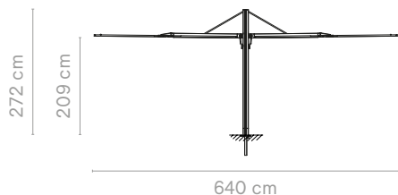
Carré duo + ancrage au sol
