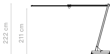
Kosmos shade carré + socle en béton à roulettes
