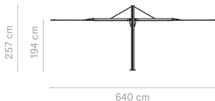
Carré duo + ancrage au sol & l'extension du mât
