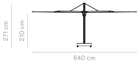
Carré duo + socle à roulettes
