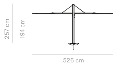
Diamant quattro + fixation permanente & l'extension du mât
