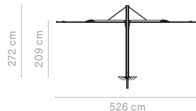
Diamant quattro + ancrage au sol
