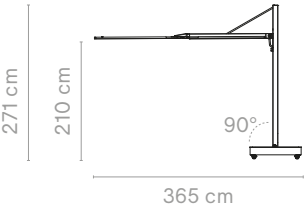
Carré simple straight + socle à roulettes
