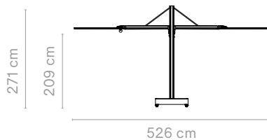
Diamant duo + socle à roulettes
