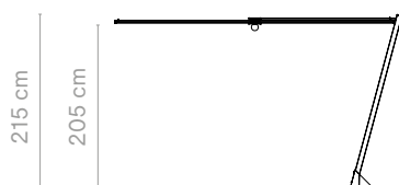
Kosmos shade carré haute + ancrage au sol
